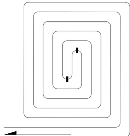
Installation of EUROTOP Mini mats.
